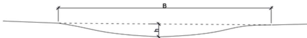
Obr. 1-44. Vzorový řez – Parabolický profil stabilizované dráhy soustředěného odtoku
