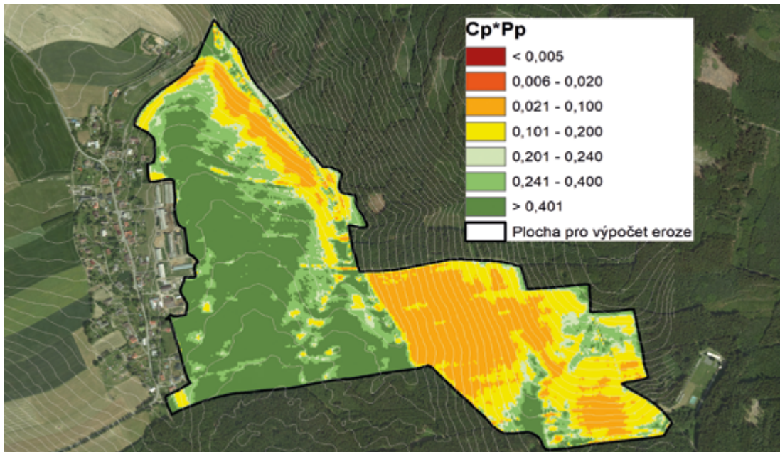
Obr. 6-10. Ukázka stanovení urstvy C_p \cdot P_p pro modelové území
