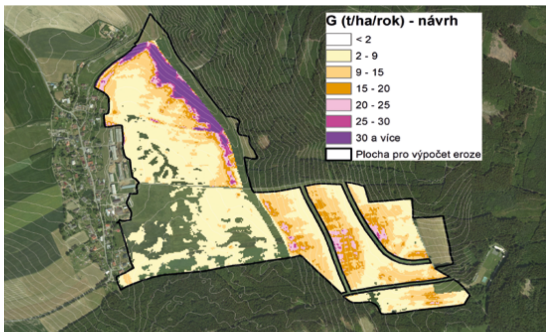
Obr. 6-15. Ukázka vypočtené vrstvy dlouhodobé průměrné ztráty půdy vodní erozí „ G “ po návrhu TPEO v modelovém
