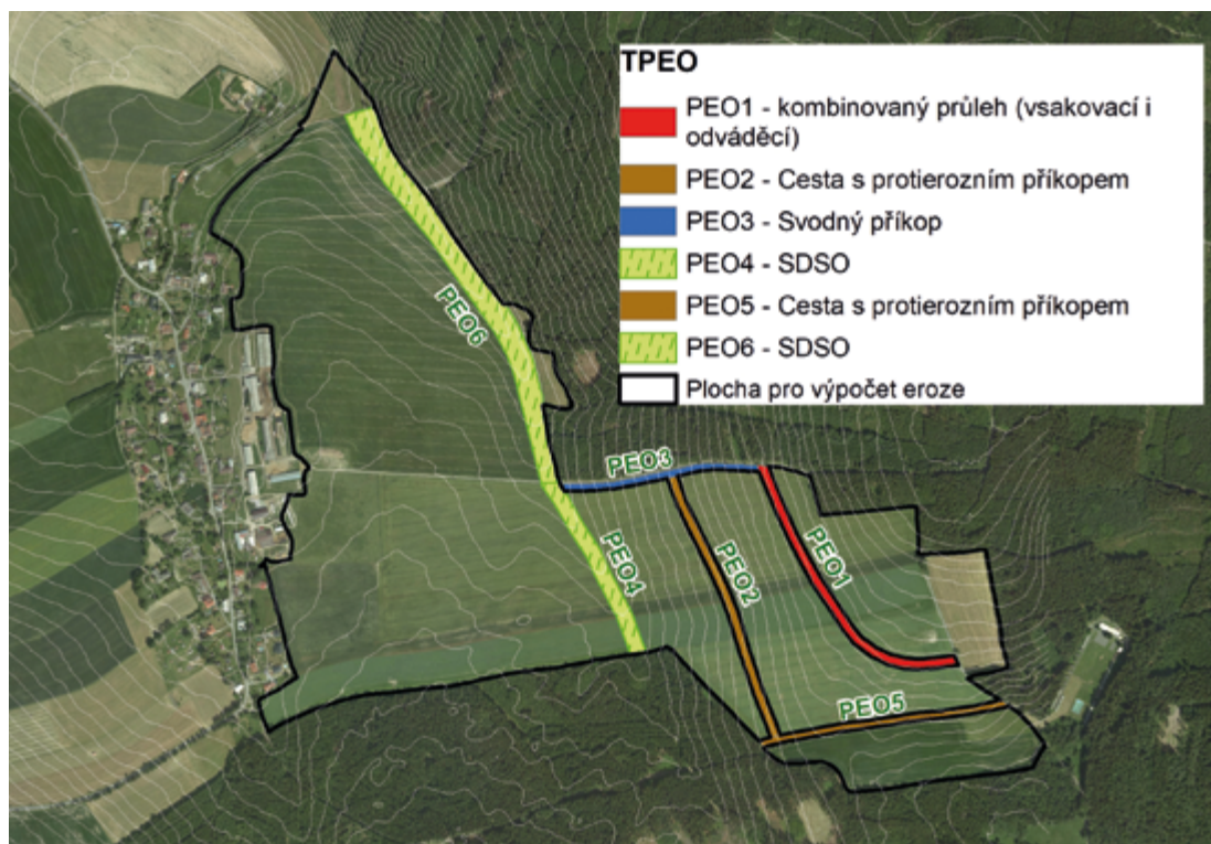
Obr. 6-13. Ukázka návrhu technických protierozních opatření (TPEO) v modelovém území
