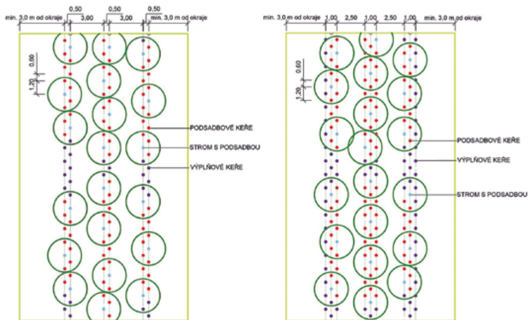
Obr. 3-13. Výsadbové schéma využívající systém dvouřad (ulevo) a výsadbové schéma využívající systém trojřad (upravo)
