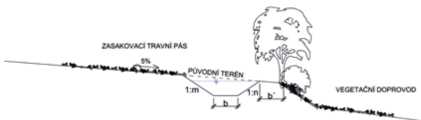
Obr. 1-34. Vzorový řez – Mez kombinovaná (vsakovací + odváděcí funkce) s liniovým prvkem (příkop) nad mezí, se zasakovacím travním pásem a s vegetačním doprovodem
