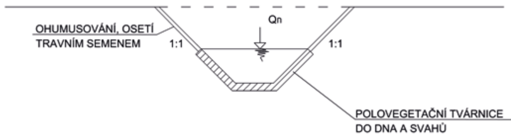
Obr. 1-48. Vzorový řez – Zpevnění svodného příkopu polovegetačními tvárnici
