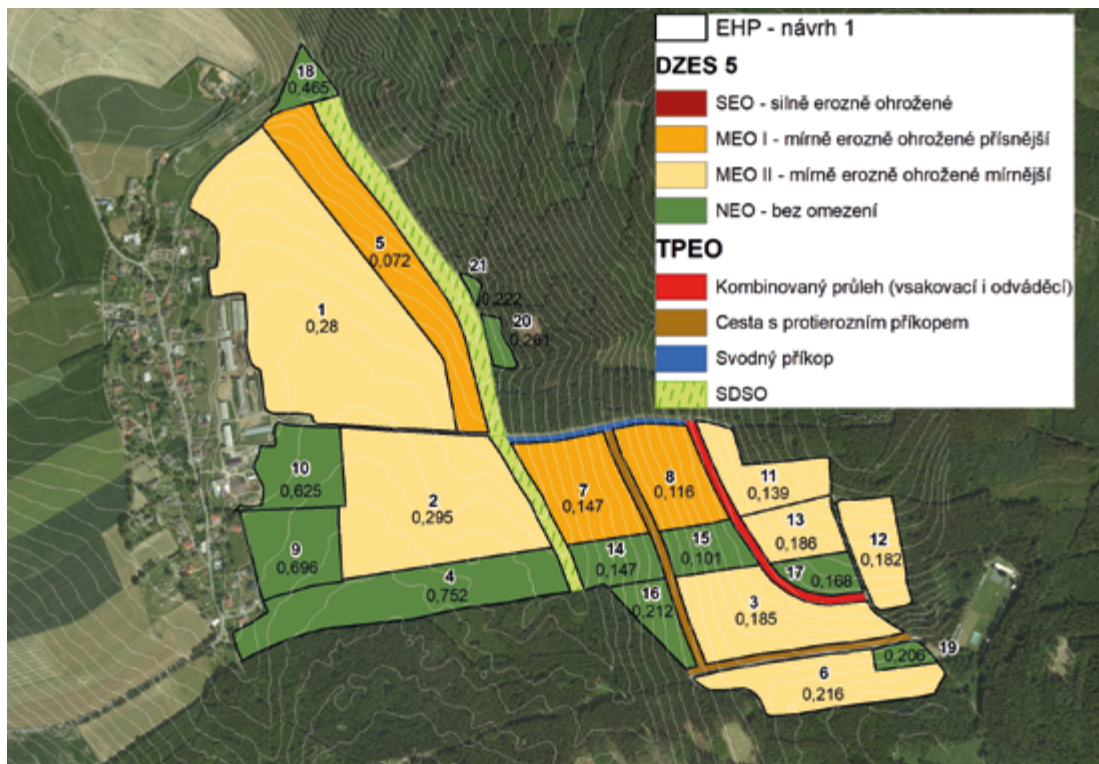
Obr. 6-19. Ukázka výsledného řešení návrhu TPEO v kombinaci s limitními hodnotami C_p \cdot P_p u modelovém území (varianta EHP – návrh 1).
