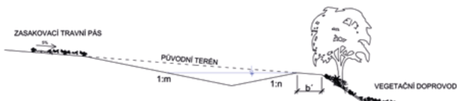
Obr. 1-35. Vzorový řez – Mez kombinovaná (vsakovací + odváděcí funkce) s liniovým prvkem (průleh) nad mezí, se zasakovacím travním pásem a s vegetačním doprovodem
