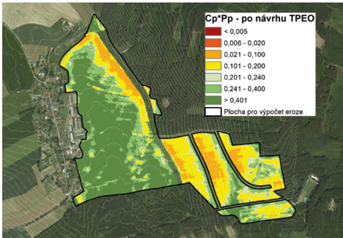
Obr. 6-18. Ukázka stanovení C_p \cdot P_p po návrhu technických/biotechnických protierozních opatření v modelovém území
