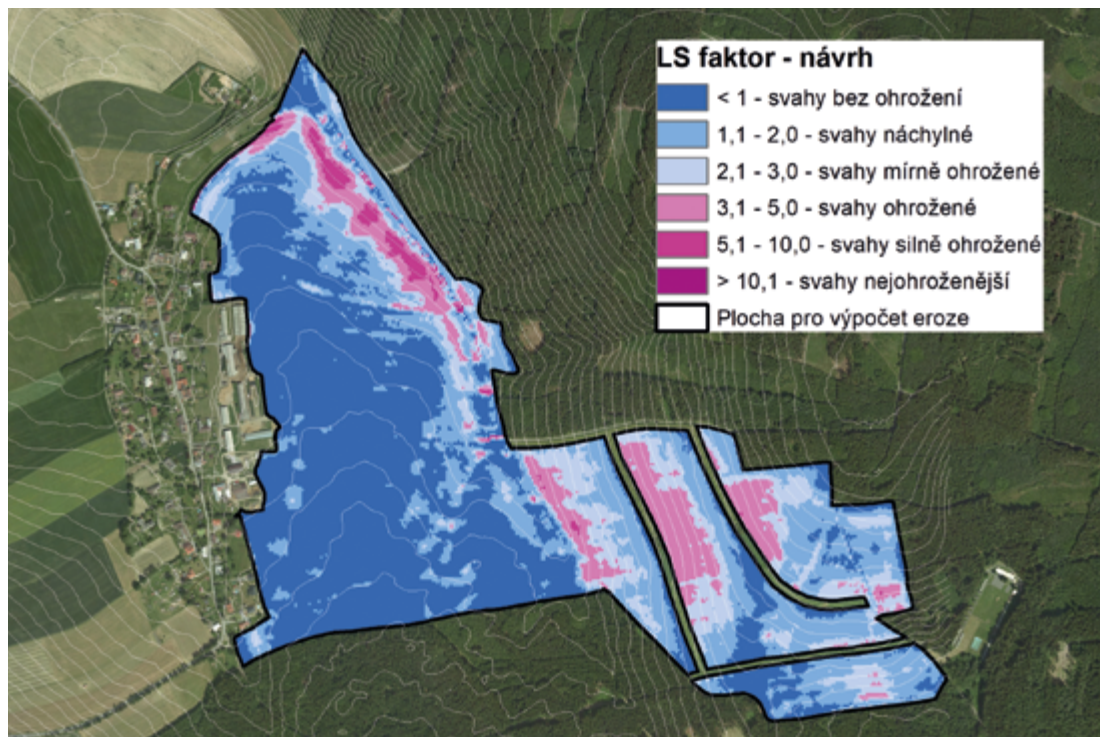
Obr. 6-14. Ukázka stanovení LS faktoru po návrhu TPEO v modelovém území
