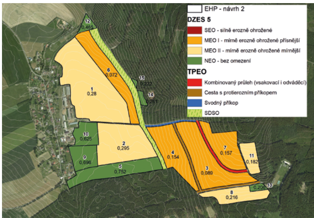
Obr. 6-20. Ukázka výsledného řešení návrhu TPEO v kombinaci s limitními hodnotami C_p \cdot P_p u modelovém území (varianta EHP – návrh 2)
