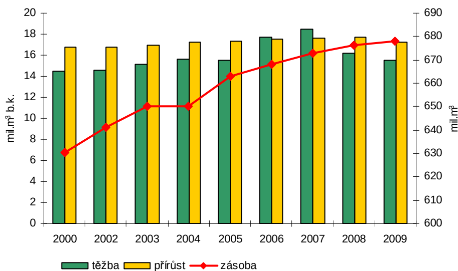
Graf 3 Porovnání celkového průměrného přírůstu s realizovanými těžbami dřeva [mil. m 3 b.k.] a celkovými porostními zásobami v ČR [mil. m 3 ], 2000–2009
