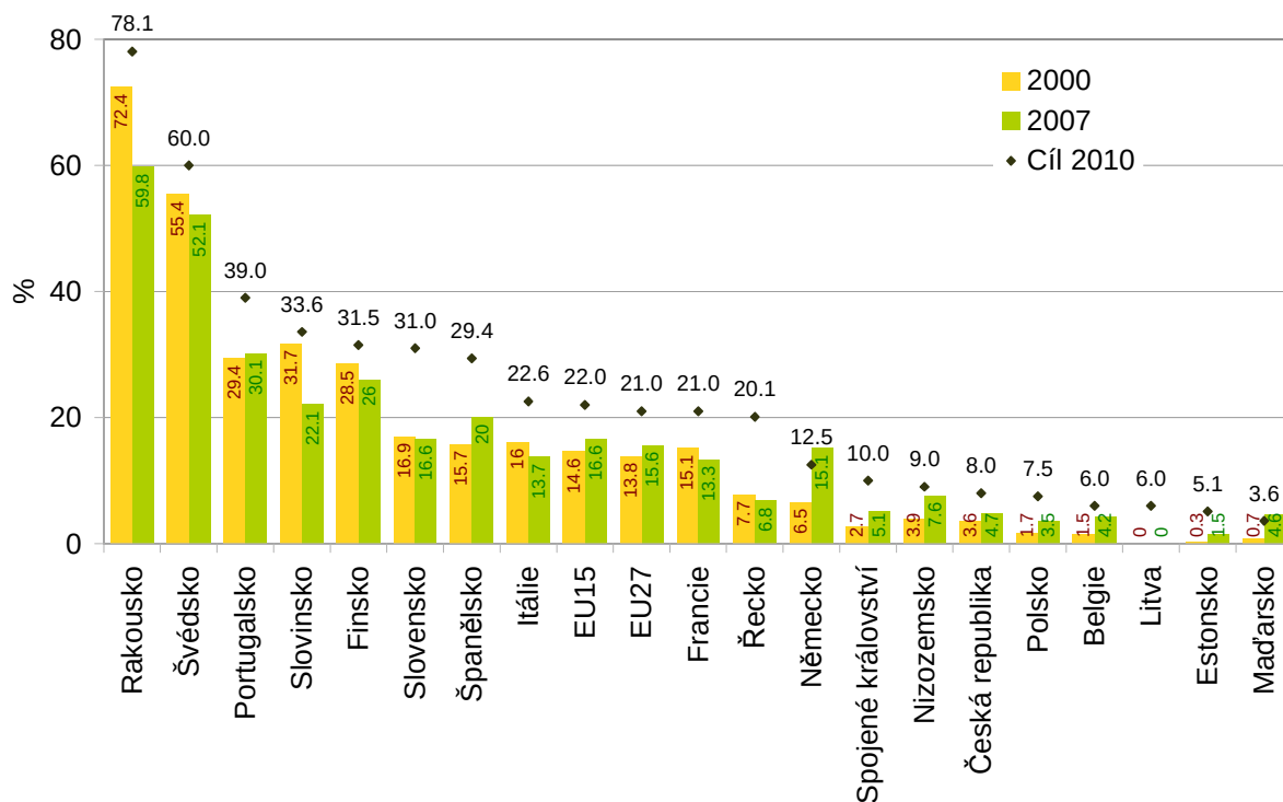
Graf 4 Mezinárodní srovnání podílu obnovitelných zdrojů energie na hrubé spotřebě elektriny [%], 2000, 2007
