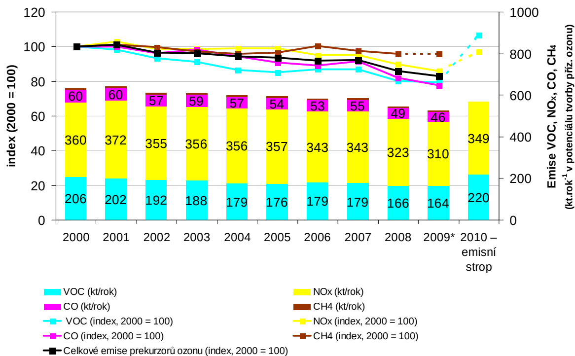
Graf 1 Vývoj celkových emisí prekurzorů ozonu v ČR, 2000–2009* a úrovně národních emisních stropů (pro VOC a NO x ) pro rok 2010 [index, 2000 = 100 (levá osa)]; [kt.rok -1 v potenciálu tvorby přízemního ozonu (pravá osa)]
