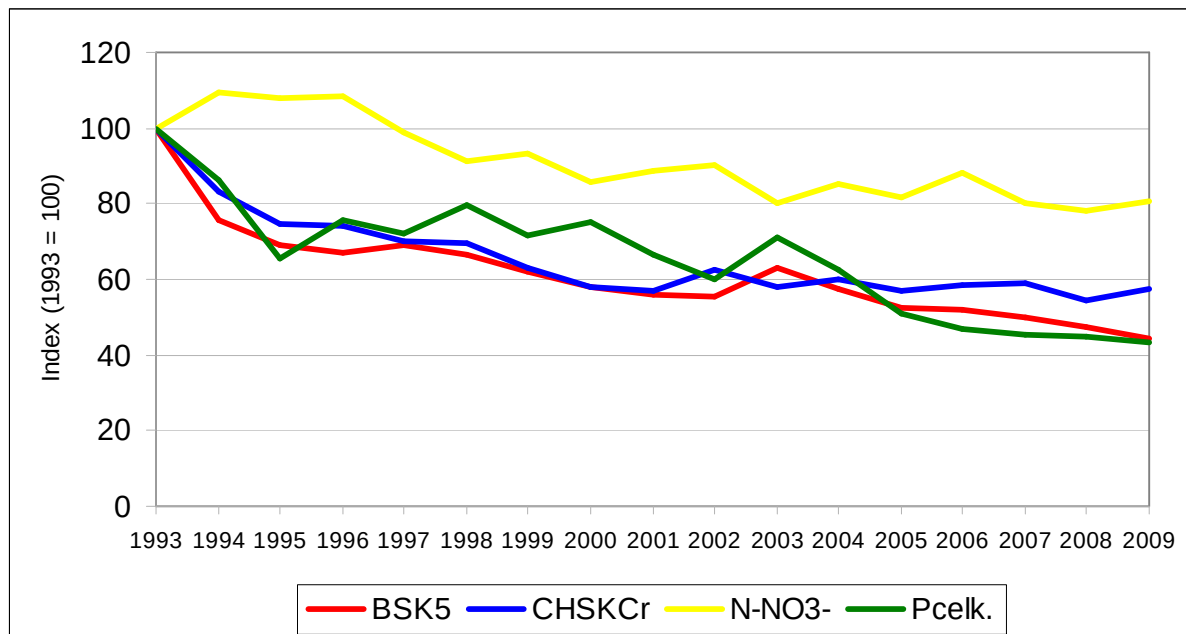
Graf 2 Vývoj koncentrací ukazatelů znečištění ve vodních tocích ČR [index, 1993 = 100], 1993–2009
