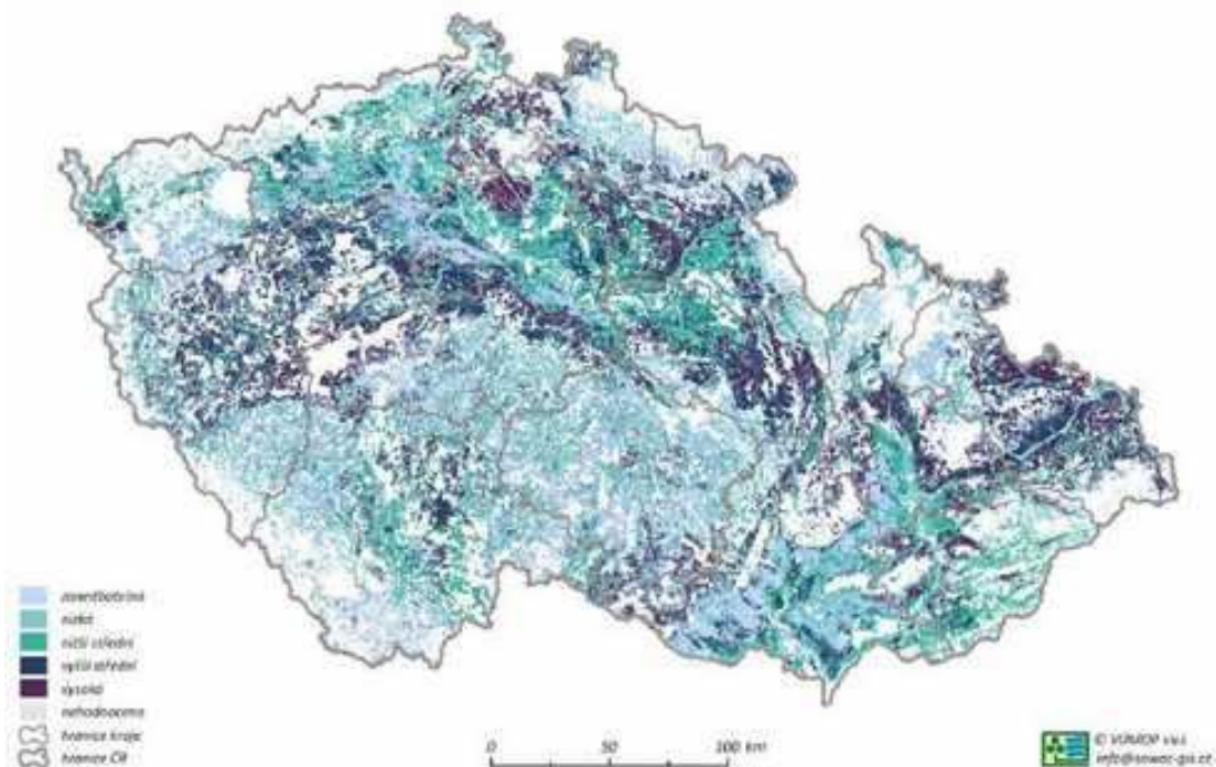
Obr. 2 Potenciální zranitelnost spodních vrstev půdy utužením, 2009
