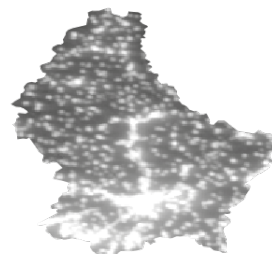
Fig. 41: Luxembourg’s night lights
