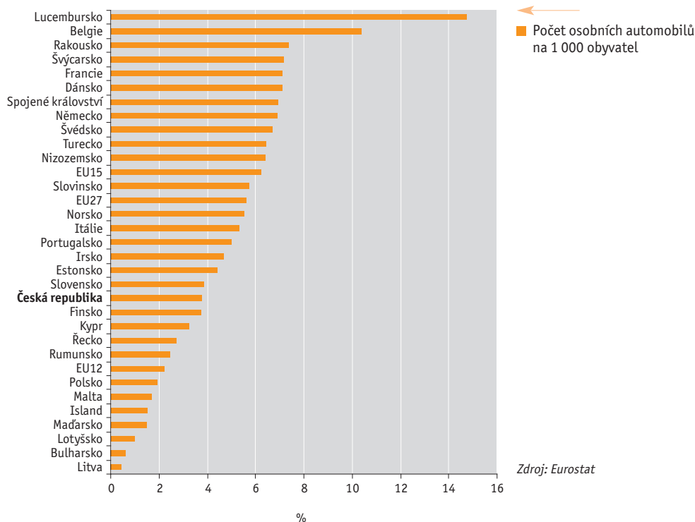
Graf 4 → Koefficient obměny vozového parku osobních automobilů [%], 2010
